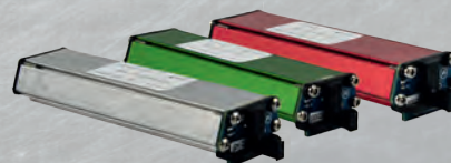
Von links nach rechts: Kältemittelsensor 724-701-G1, CO 2 -Sensor 724-701-G2 und Sensor für brennbare Kältemittel 724-701-G3.
